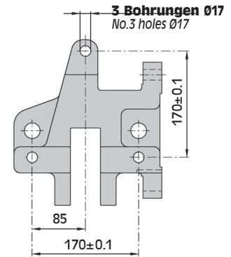
Front Ansicht Anschraubfläche Frontal mounting view
